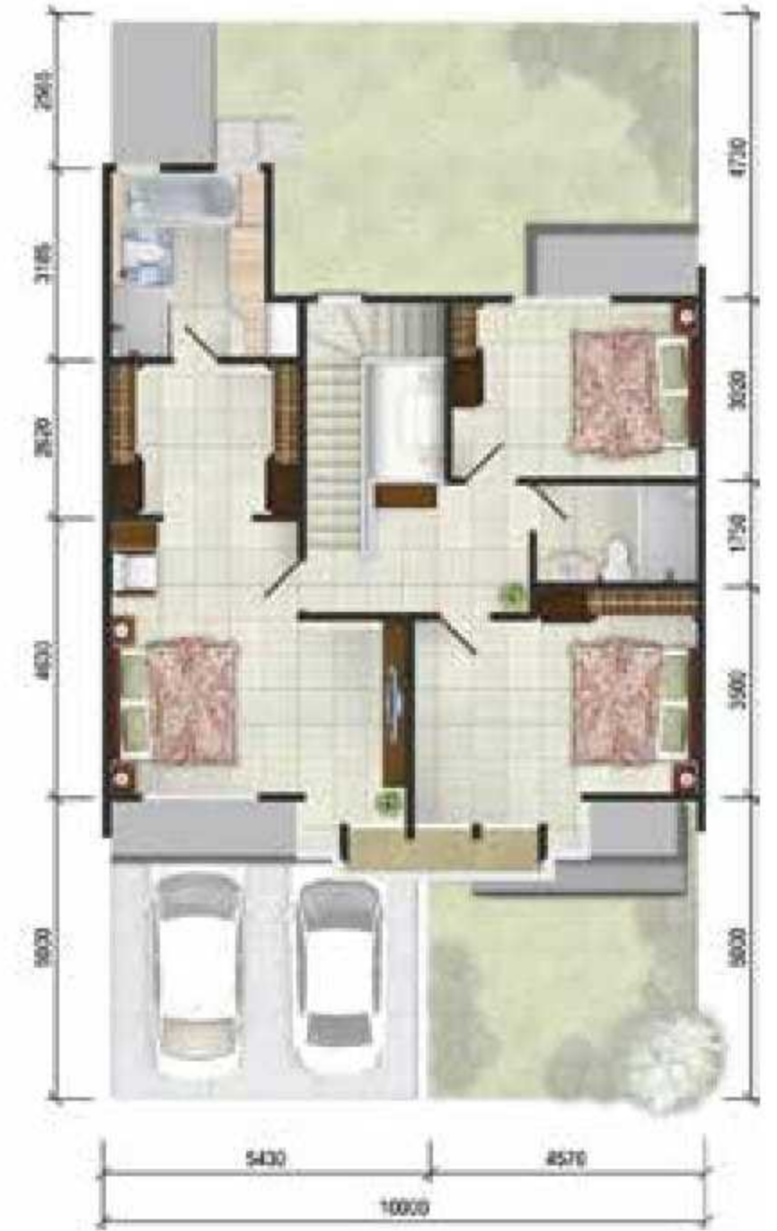
LANTAI ATAS
