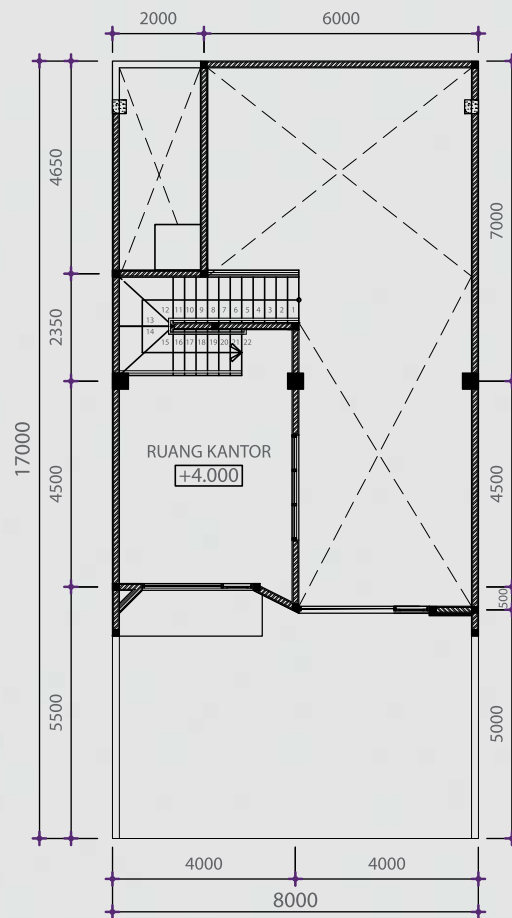
LANTAI ATAS
