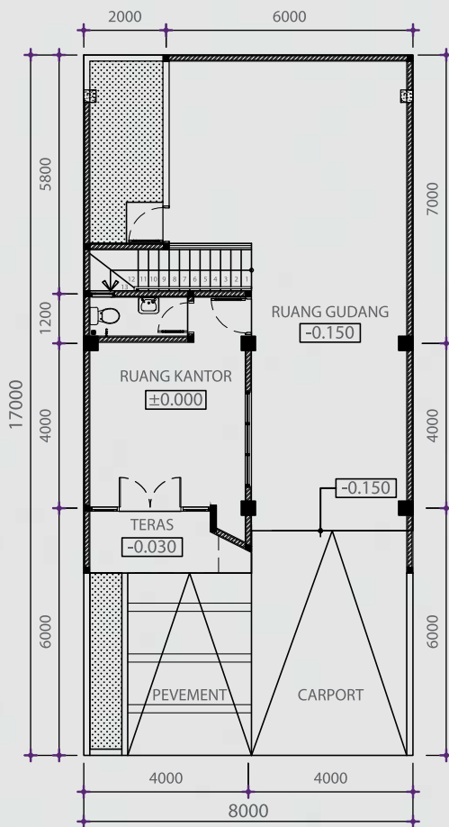
LANTAI DASAR
