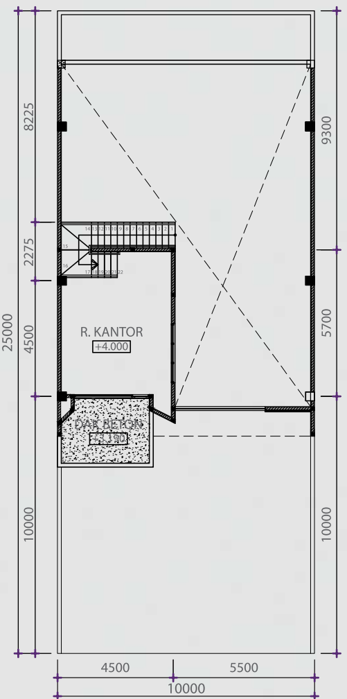
LANTAI ATAS
