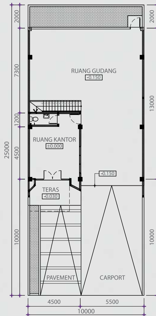
LANTAI DASAR
