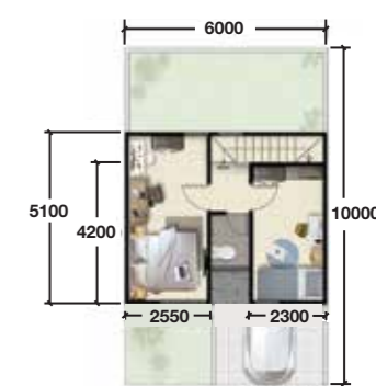
Lantai 2
