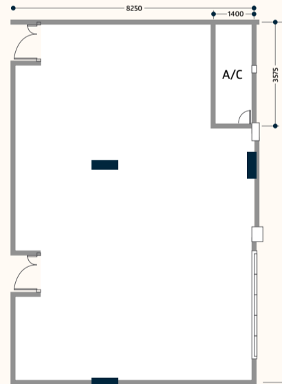
Type F1 Floor Area : 1109 sq. ft. Location : Block B First Floor
