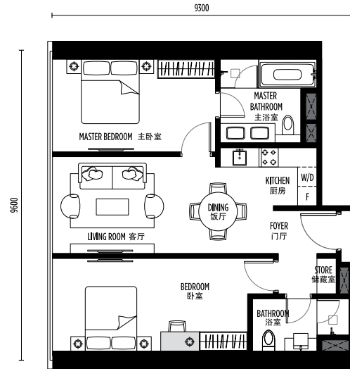
TYPE D-1 户型 2 BEDROOMS 房 84 SQ.M. 平方米 / 903 SQ.FT. 平方英尺
