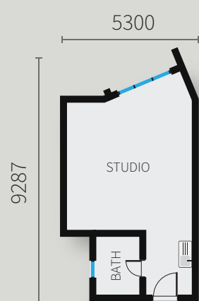
A1 452 sq. ft
