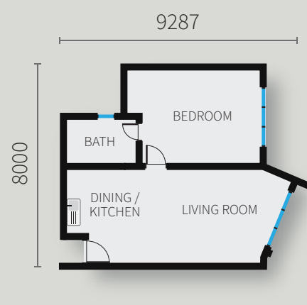
B3 646 sq. ft
